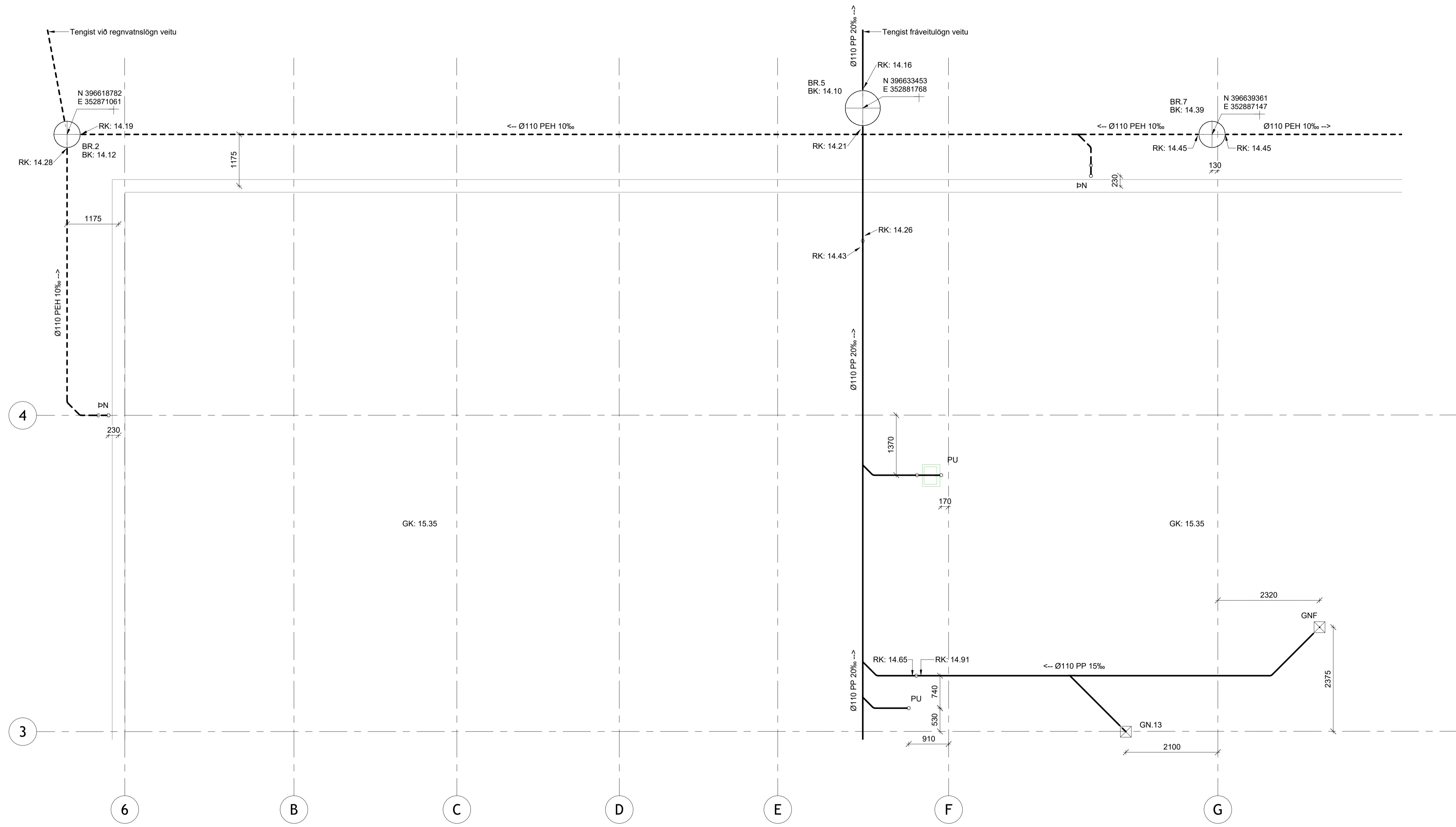
Grunnmynd 1 af 4 1 : 50
