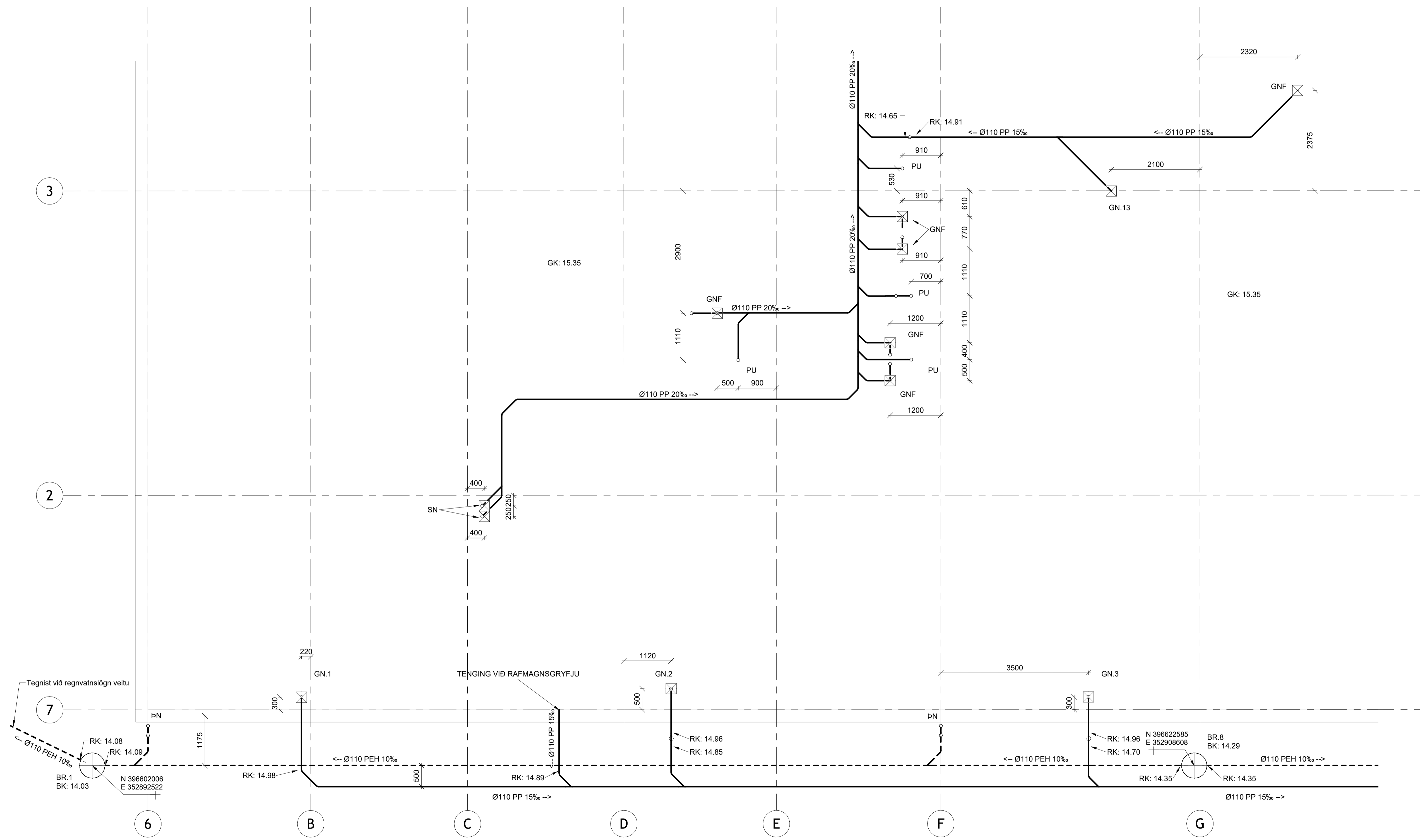
Grunnmynd 3 af 4 1 : 50
